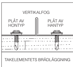
Detalj 1:2
