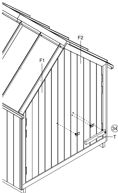
Detaljritning för festsättning av trådhake
