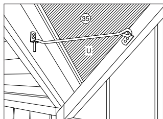
Detaljritning för festsättning av trådhake
