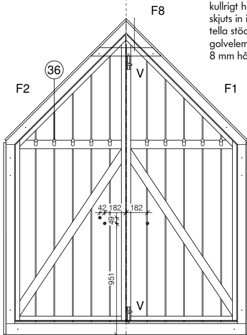
Projektionsbild av gavelementen bakifrån
