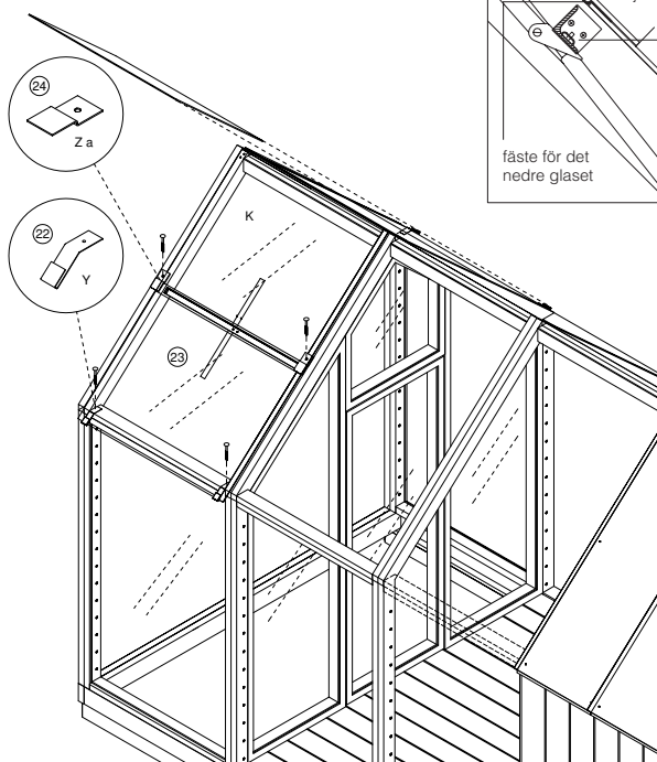
Detalj 1:5
