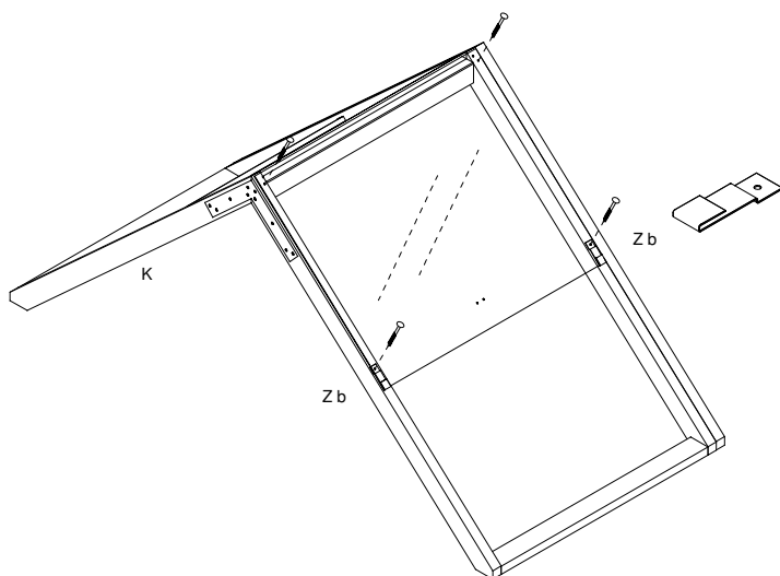
Detalj: fastsättning av glas
