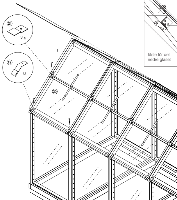
Detalj 1:5
