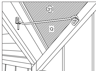
Detaljritning för fastsättning av trådhooken.
