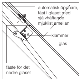
Detalj 1:5
