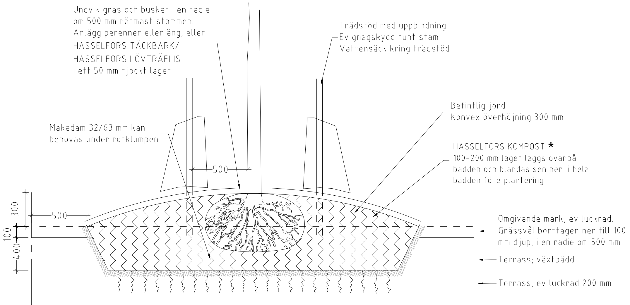
TRÄD: VÄXTBÄDD TYP 3 MED JORDFÖRBÄTTRING LERIGA FÖRHÅLLANDEN PRINCIPSEKTION SKALA 1:20/A1. Alla mått i mm Uppbyggnad enl. AMA DCL.121 och DCL.412
