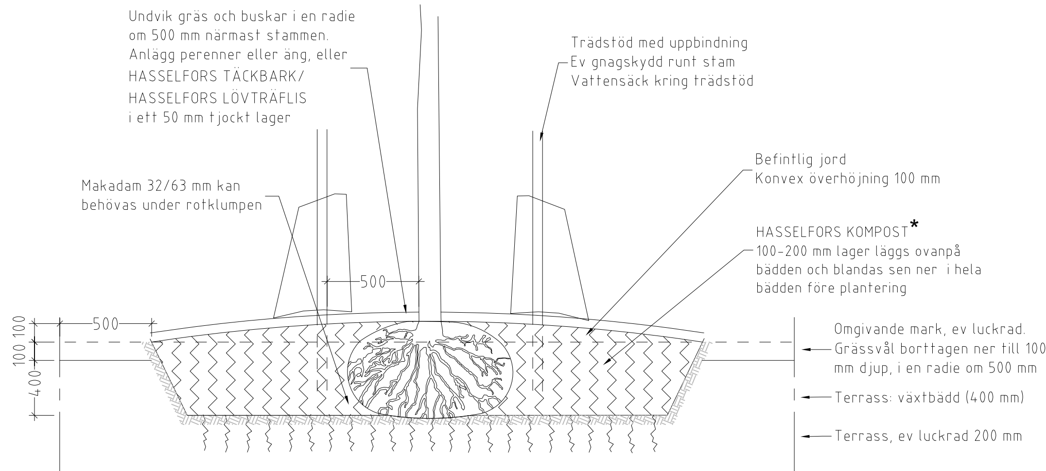
TRÄD: VÄXTBÄDD TYP 3 MED JORDFÖRBÄTTRING ICKE LERIGA FÖRHÅLLANDEN PRINCIPSEKTION SKALA 1:20/A1. Alla mått i mm Uppbyggnad enl. AMA DCL.121 och DCL.412
